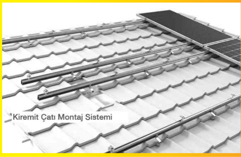
Kiremit Çatı Konstrüksiyonu
